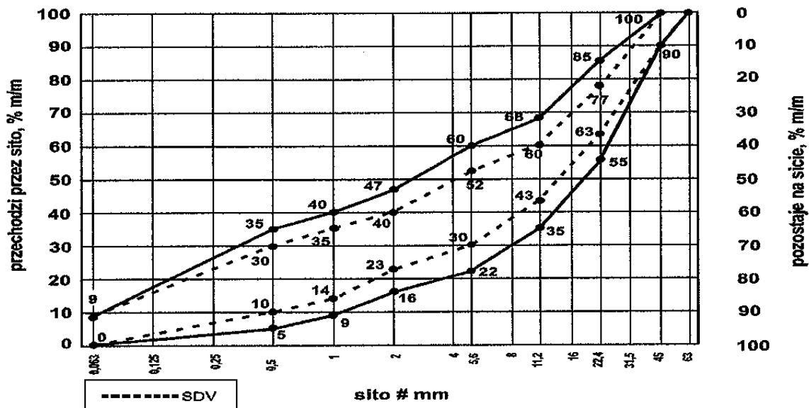
Tablica 4. Wymagania wobec mieszanek kruszywa niezwiązanego w warstwie podbudowy zasadniczej
