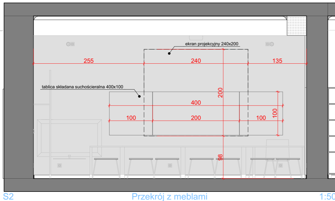
S2 Przekrój 1:50
