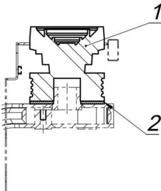
nr 2 – element gumowo-metalowy usprężynowania II stopnia.
