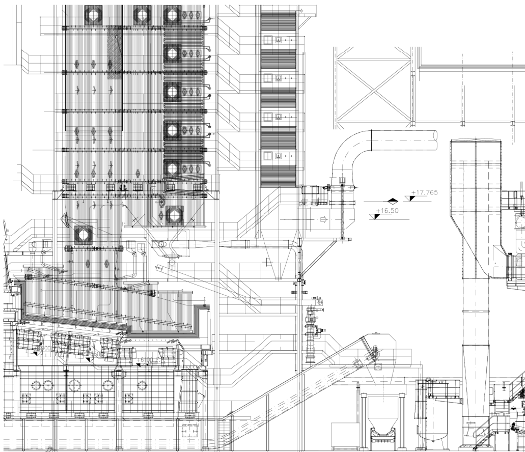
PRZEKROJE "B-B" (SECTION "B-B")
