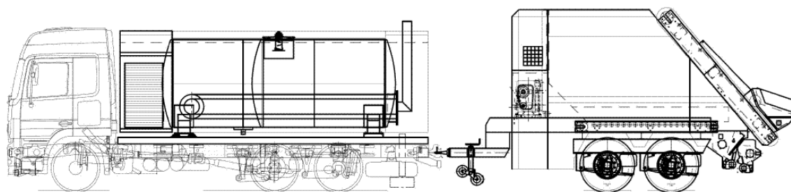
Rys. 4. Schemat kombajnu drogowego do powierzchniowego utwalenia nawierzchni ( http://www.asphalt.de/media/Flyer_-_Prospekte/AS_GmbH_-_Prospekt_OB.pdf )
