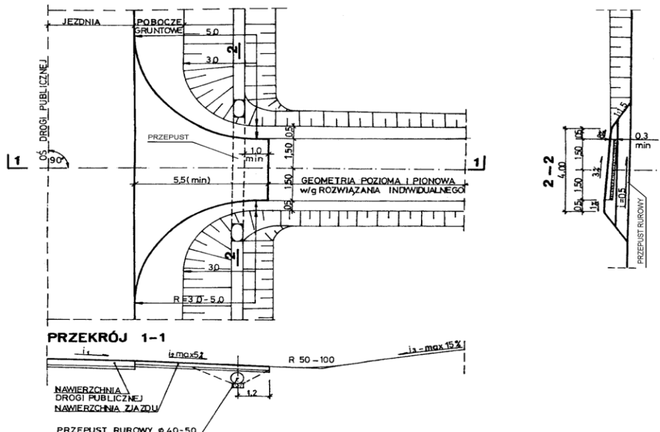
Rys. 3.1. Przykładowe rozwiązanie sytuacyjne zjazdu indywidualnego z przepustem
