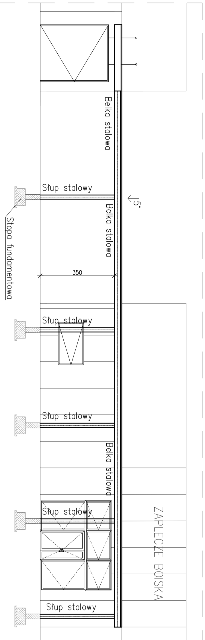
PRZEKRÓJ/WIDOK ZADASZENIA SKALA 1:100
