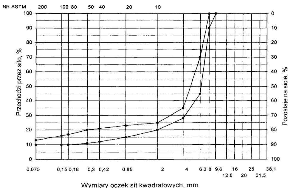
Rys. 7. Krzywe graniczne uziarnienia mieszanki mineralnej SMA od 0 do 8 mm do warstwy ścieralnej nawierzchni drogi
