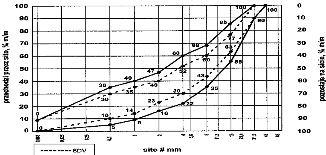
Rys. 1. Krzywe graniczne uziarnienia mieszanki kruszywa niezwiązanego 0/31,5 mm do warstw nawierzchni
