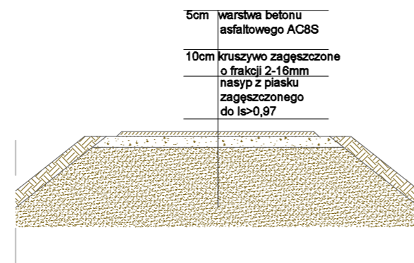
Przekrój poprzeczny toru pump tracku SKALA 1:50
