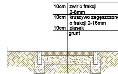
Przekrój poprzeczny ścieżki żwirowej na wysokości +3,00m SKALA 1:50
