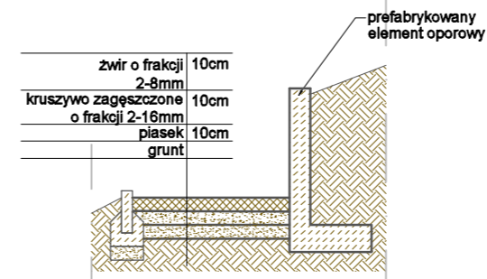
Przekrój poprzeczny ścieżki żwirowej na wysokości +4,90m SKALA 1:50
