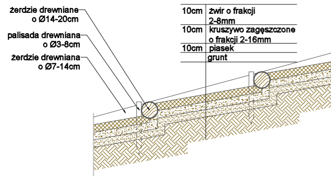
Przekrój podłużny ścieżki z bali SKALA 1:50
