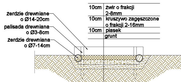
Przekrój poprzeczny ścieżki z bali SKALA 1:50
