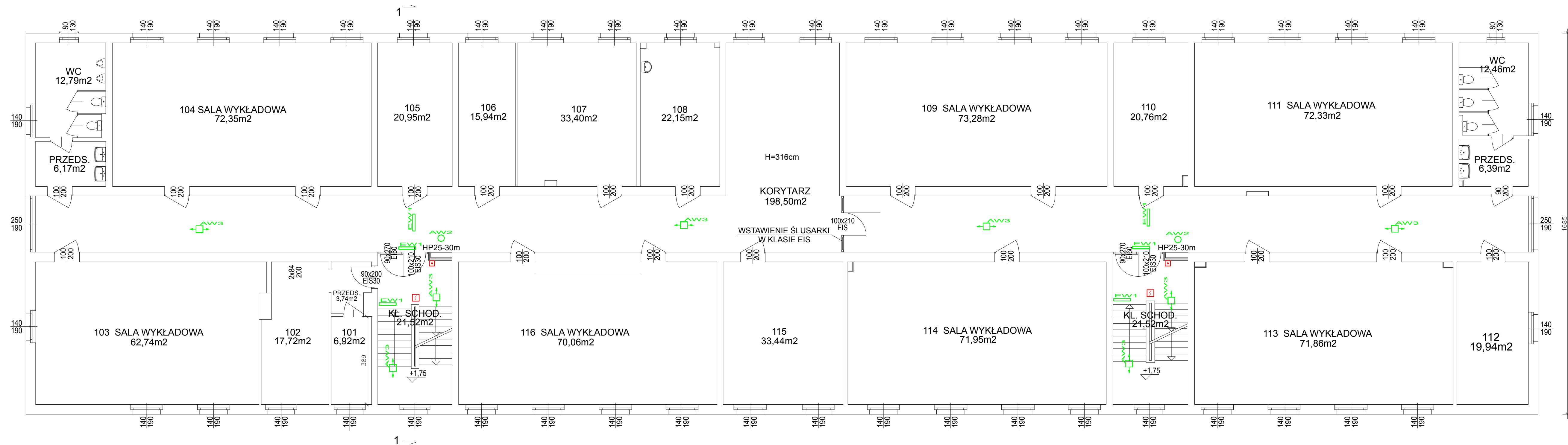
RZUT I PIĘTRA - STAN PROJEKTOWANY 1:100 BUDYNEK "B"
