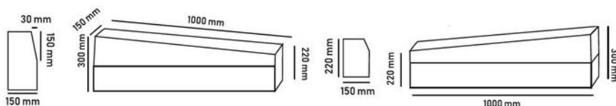
b) krawężnik skośny
