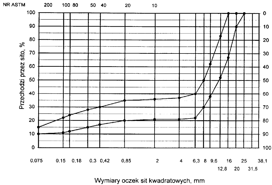
Rys. 5. Krzywe graniczne uziarnienia mieszanki mineralnej BA od 0 do 20 mm (mieszanka o nieciągłym uziarnieniu) do warstwy ścieralnej nawierzchni drogi o obciążeniu ruchem od KR3
