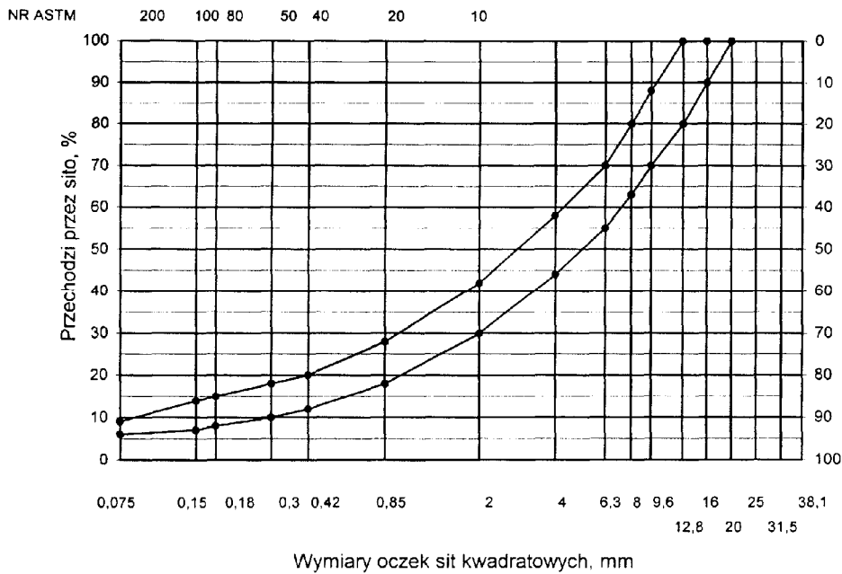
Rys. 6. Krzywe graniczne uziarnienia mieszanki mineralnej BA od 0 do 16 mm do warstwy ścieralnej nawierzchni drogi o obciążeniu ruchem od KR3
