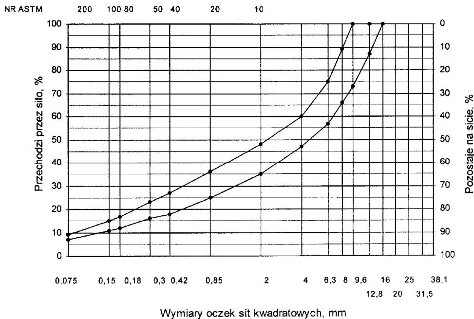
Rys. 7. Krzywe graniczne uziarnienia mieszanki mineralnej BA od 0 do 12,8 mm do warstwy ścieralnej nawierzchni drogi o obciążeniu ruchem od KR3
