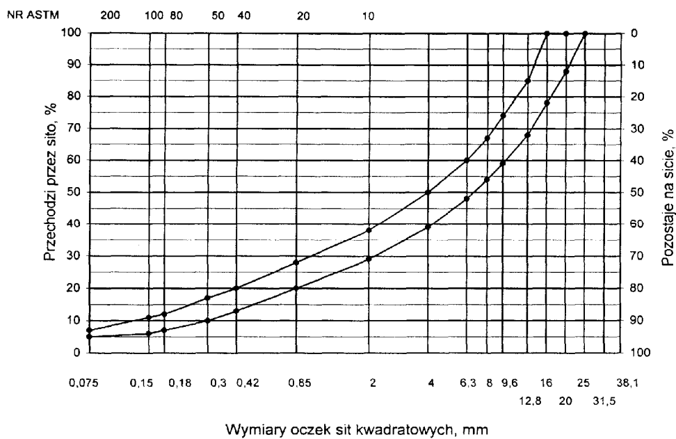
Rys. 4. Krzywe graniczne uziarnienia mieszanki mineralnej BA od 0 do 20 mm do warstwy ścieralnej nawierzchni drogi o obciążeniu ruchem od KR3
