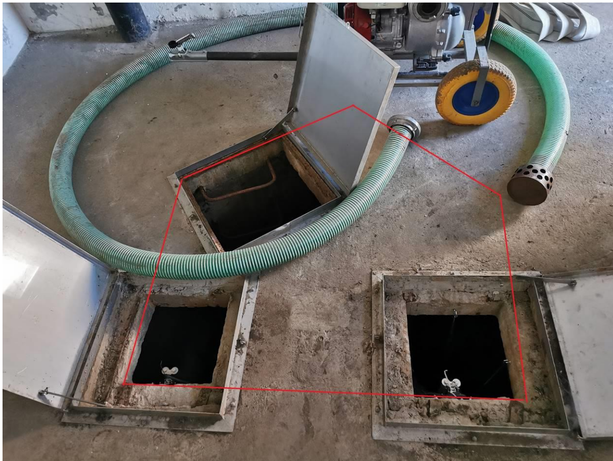
Rysunek 5. Sugerowany obszar powiększania włazów rewizyjnych
