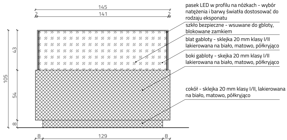
G2_3 WIDOK OD FRONTU
