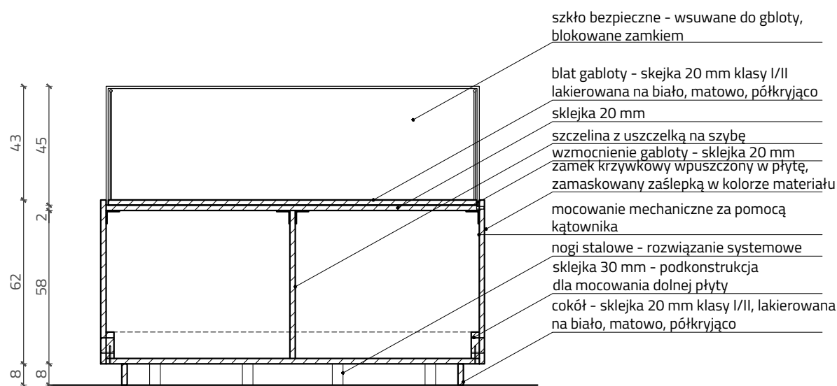
G2_3 PRZEKRÓJ PODŁUŻNY
