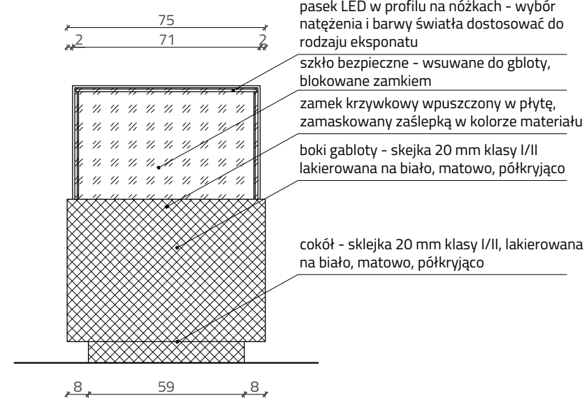
G2_3 WIDOK Z BOKU
