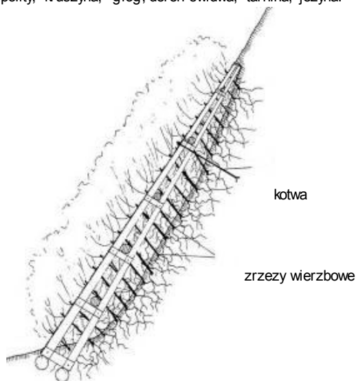
Drewniane rusztowanie na skarpie wzmocnione nasadzeniami wierzbowymi (Begemann i Schiechtel 1999)
