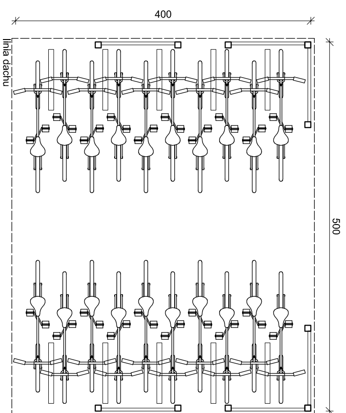
RZUT WIATY
