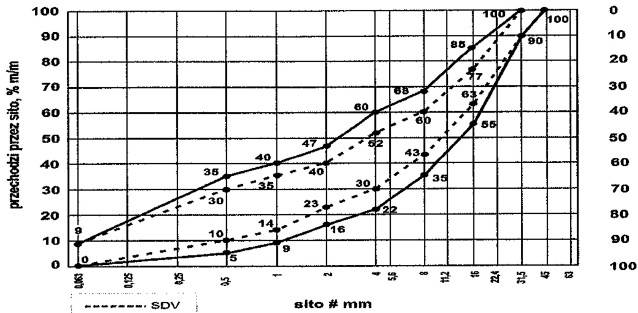
Rysunek 2. Mieszanka kruszyw 0/31,5 do górnej warstwy nawierzchni
