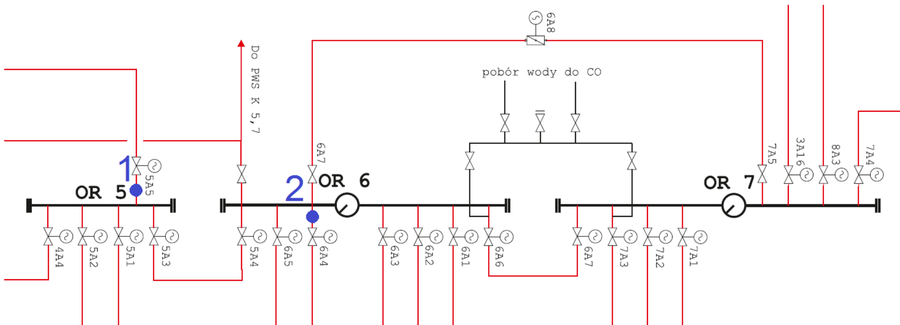
Rysunek 6 Miejsca wpięcia kotłów KRS
