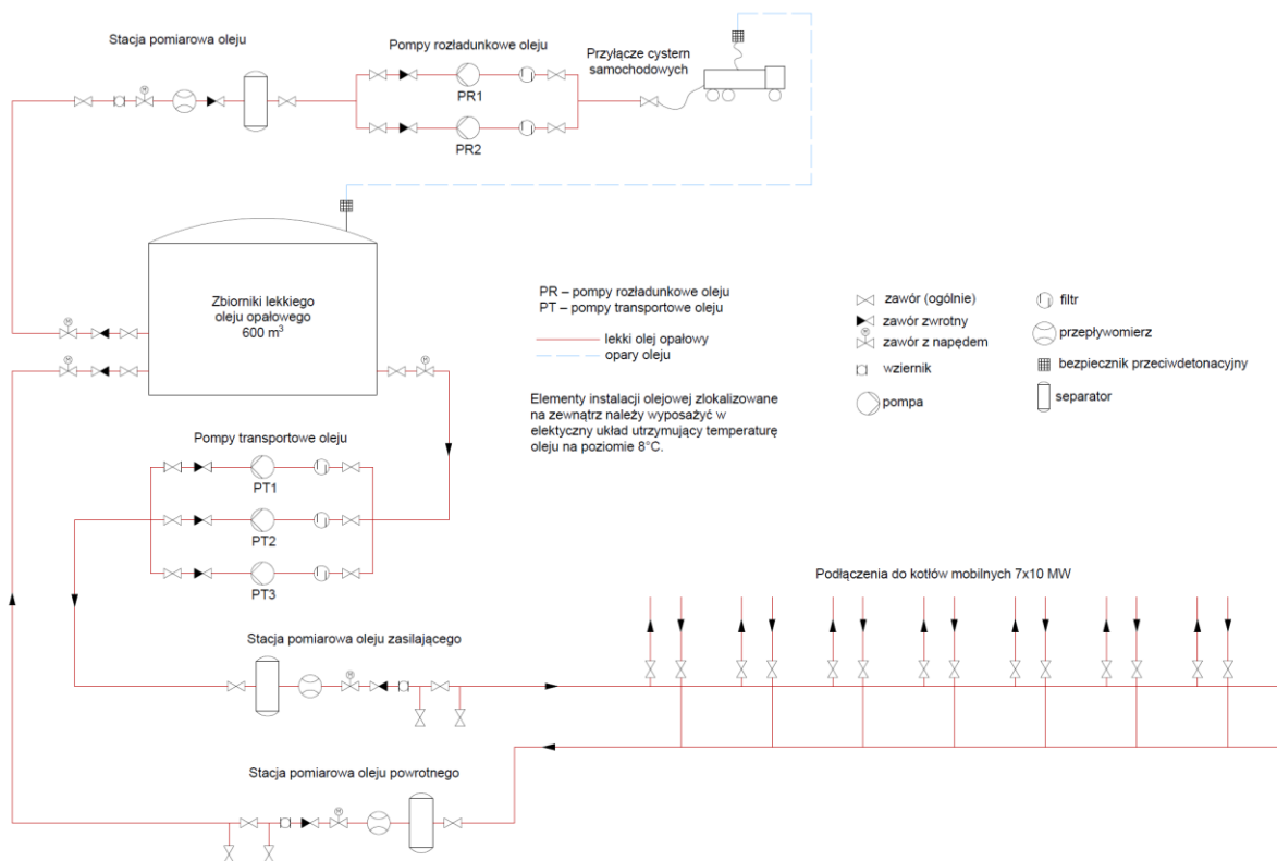
Rysunek 8 Schemat instalacji lekkiego oleju opałowego
