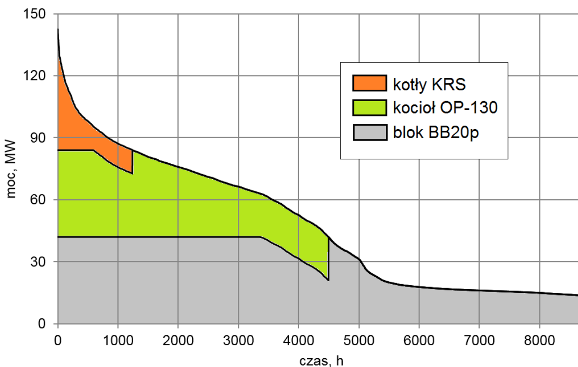
Rysunek 5 Pokrycie zapotrzebowania na produkcję ciepła
