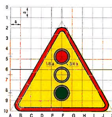
A-29 „Sygnały świetlne”
