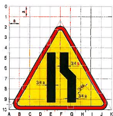
A-12b „Zwężenie jezdni - prawostronne”
