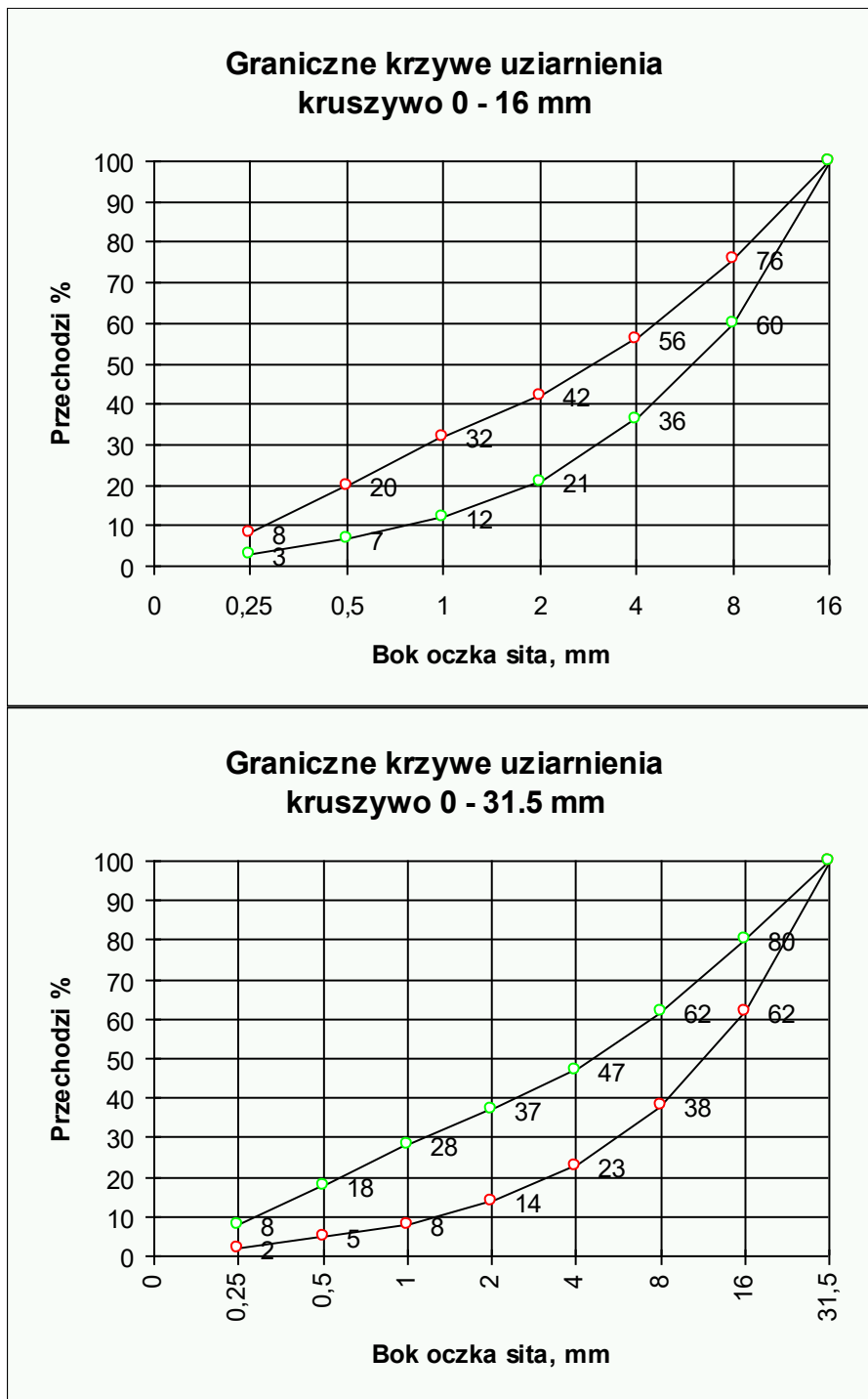
Graniczne uziarnienie kruszywa
