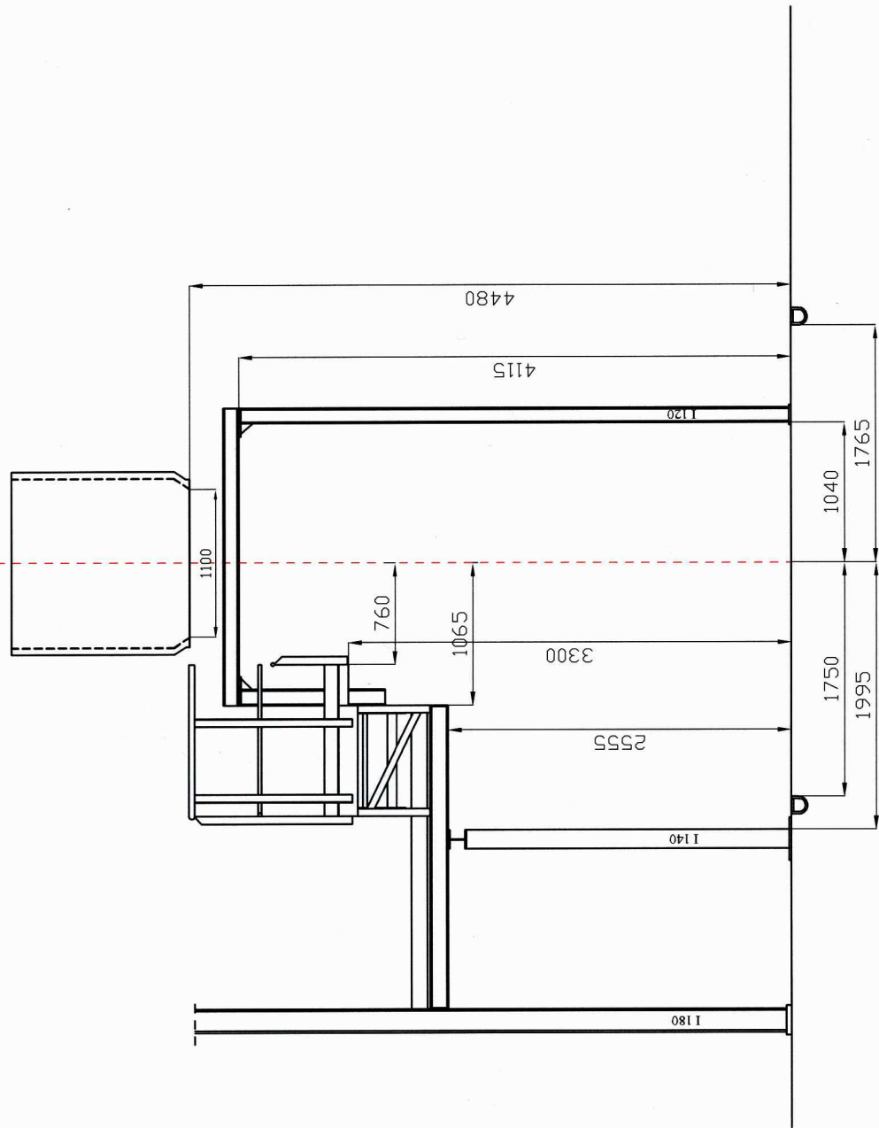
Szkic miejsca montażu prasy z rozmieszczeniem istniejących elementów linii sortowniczej rys. 1/5
