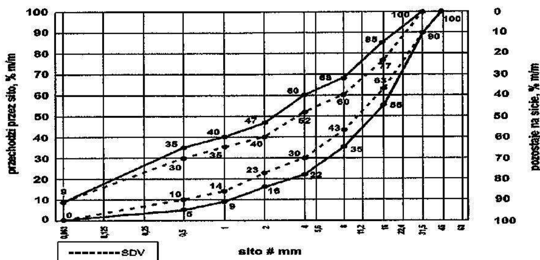
Rys. 1. Krzywe graniczne uziarnienia mieszanki kruszywa niezwiązane 0/31,5mm do warstw podbudowy
