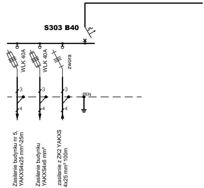
Człon kablowy
