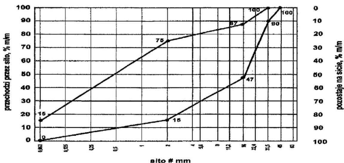
Rys. 1. Mieszanka niezwiązana 0/31,5 do wykonania pobocza
