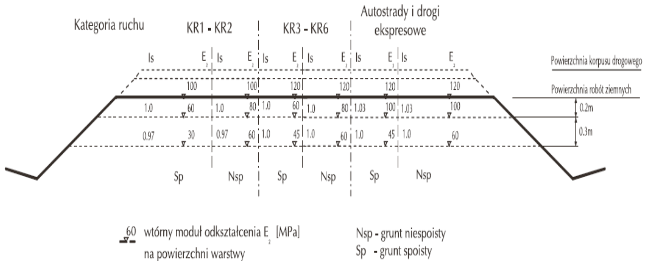
Rys. nr 1. Wymagane parametry dróg w wykopach
