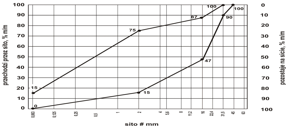
Rys. 5. Uziarnienie mieszanki niezwiązanej 0/31,5 dla warstwy mrozochronnej
