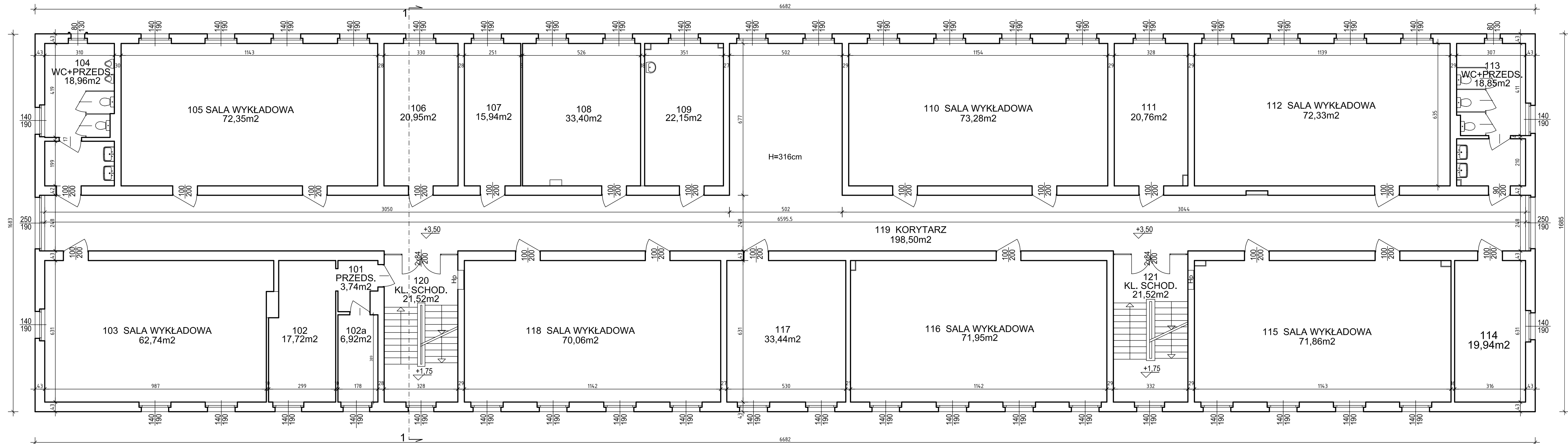
RZUT I PIĘTRA - STAN ISTNIEJĄCY 1:100 BUDYNEK "B"
