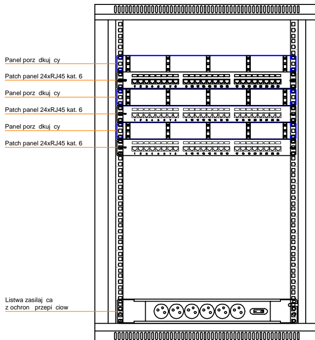
WIDOK ELEWACJI SZAFKI LPD/LAB Szafa na cienna 19"
