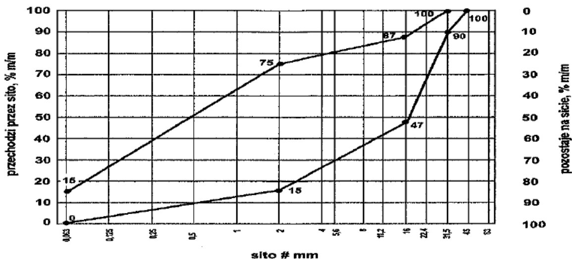
Rysunek 2. Mieszanka niezwiązana 0/31,5 do warstwy ulepszonego podłoża stabilizowanego georusztem
