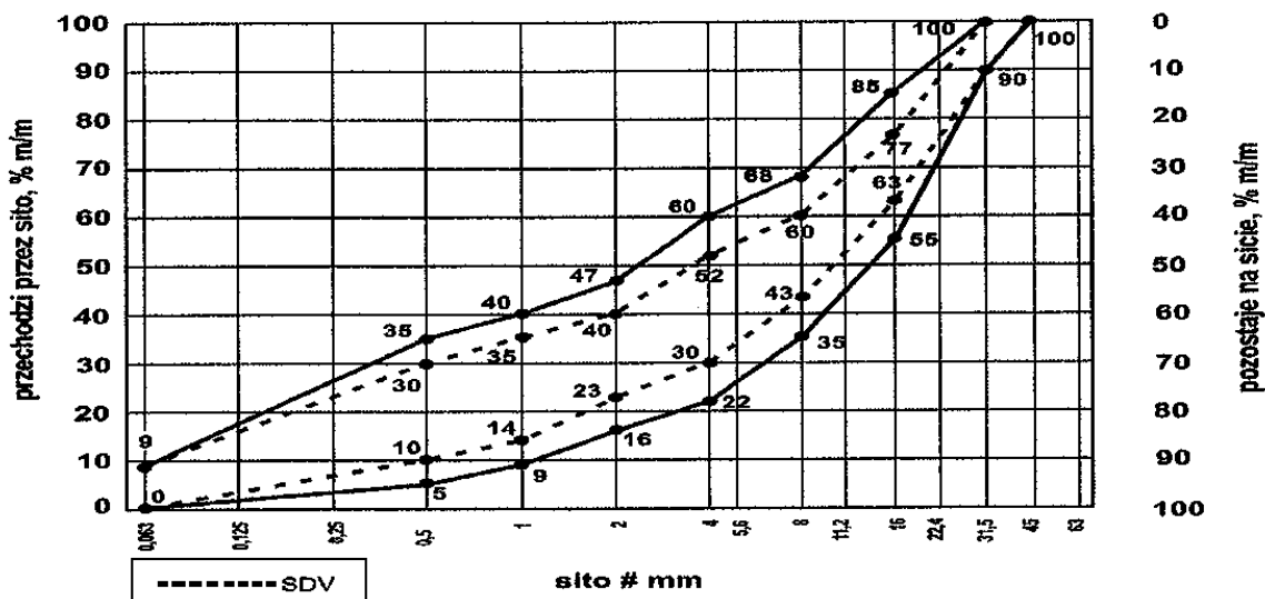
Rys 1.0 Krzywa graniczna uziarnienia mieszanki kruszywa niezwiązanego 0/31.5mm do podbudowy zasadniczej przeznaczonyj pod jezdnie oraz miejsca postojowe
