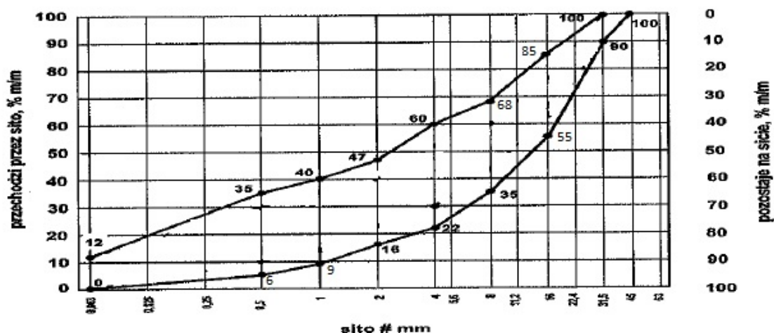
Rysunek 1. Mieszanka niezwiązana 0/31,5 do warstwy podbudowy pomocniczej stabilizowanej georusztem
