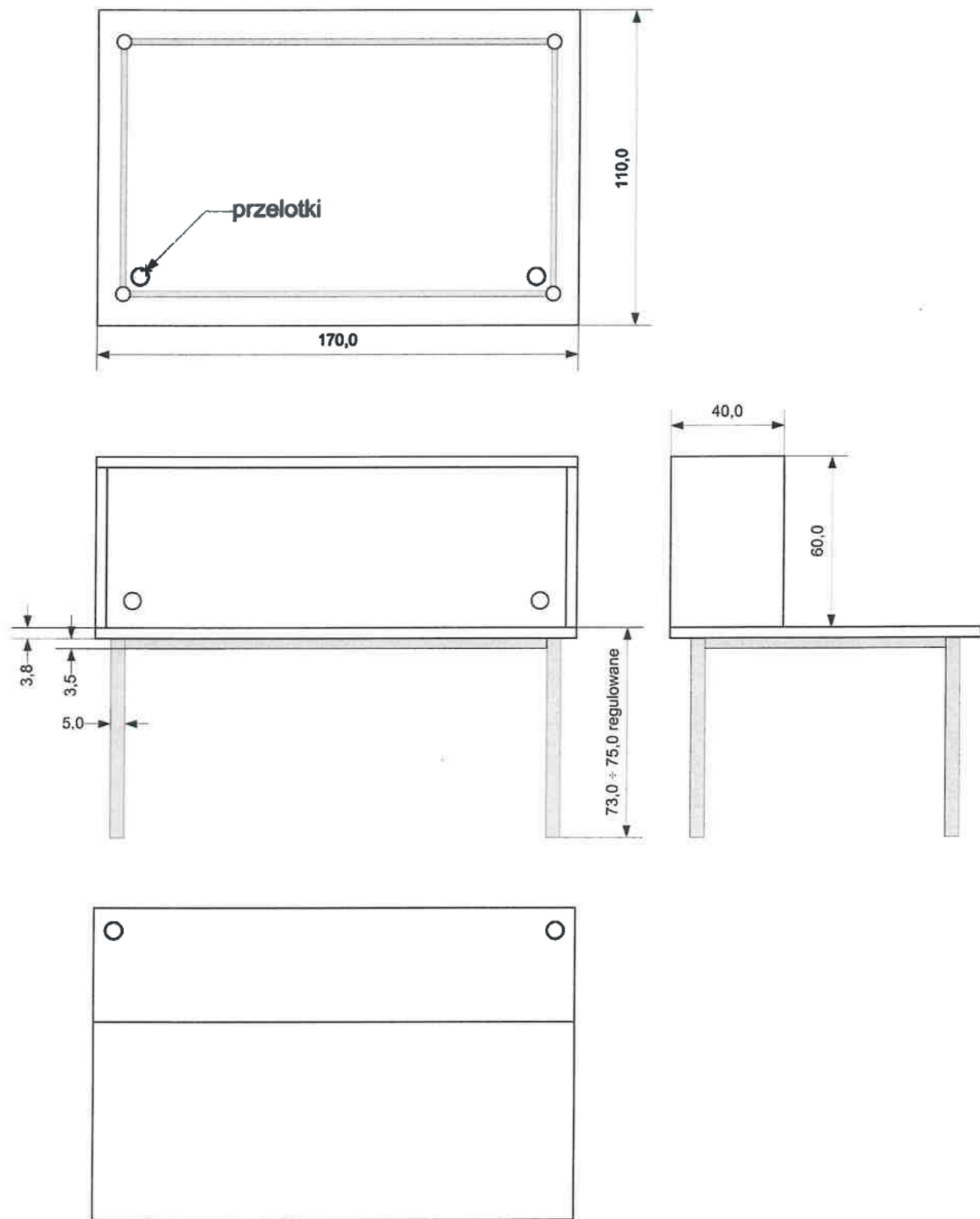
Rys. 1 Stół laboratoryjny
