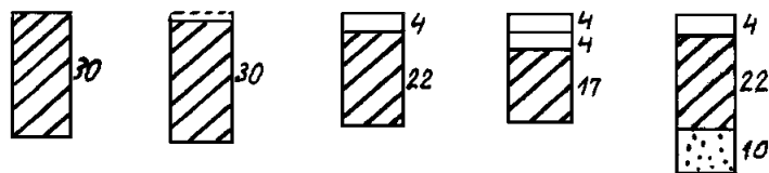
Rys. 3. Przykładowe wybrane konstrukcje nawierzchni utwardzonego pobocza z kruszywa łamanego niezwiązanego
