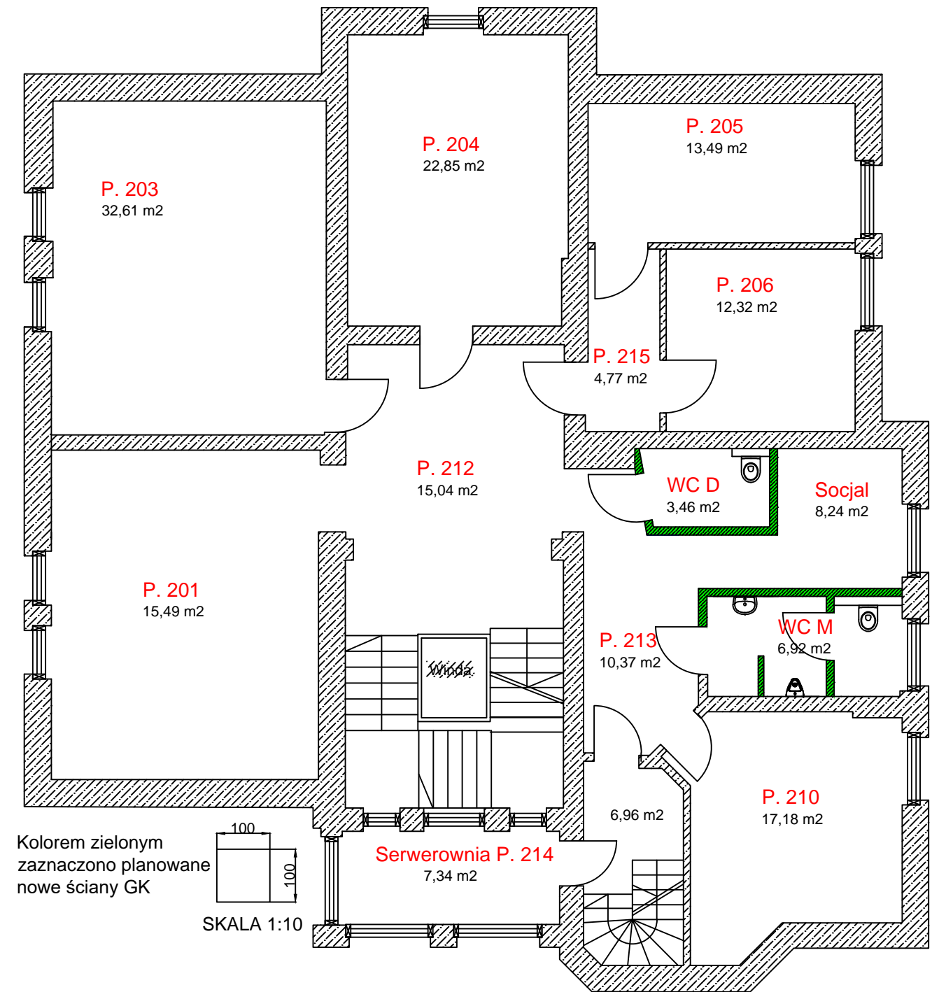
Rzut I Piętra
