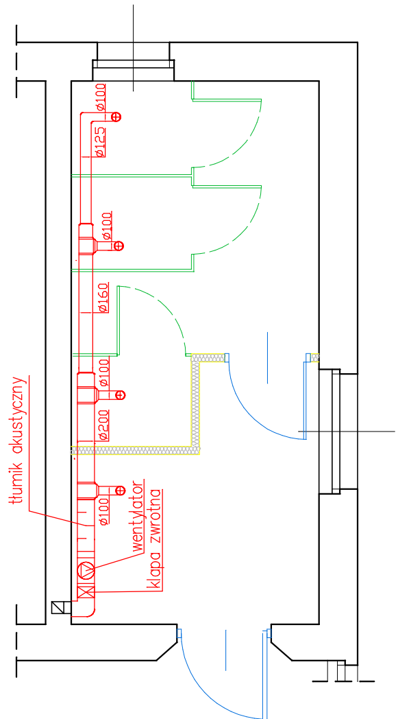
SCHEMAT WENTYLACJI WĘZŁA SANITARNEGO
