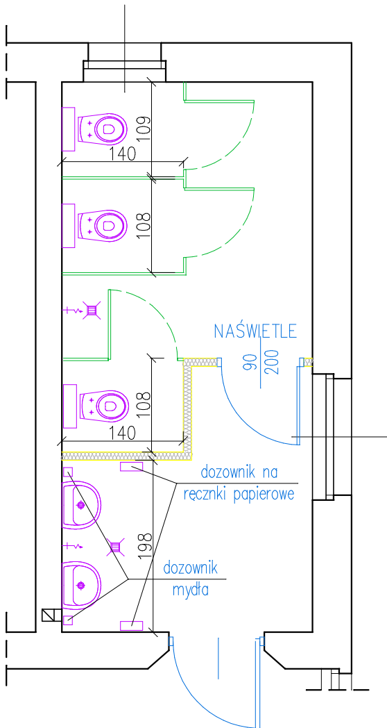
SCHEMAT WĘZŁA SANITARNEGO
