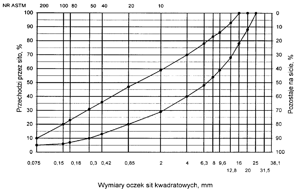
Rys. 1. Krzywe graniczne uziarnienia mieszanki mineralnej BA od 0 do 20 mm do warstwy ścierniczej nawierzchni drogi o obciążeniu ruchem dla KR1 lub KR2
