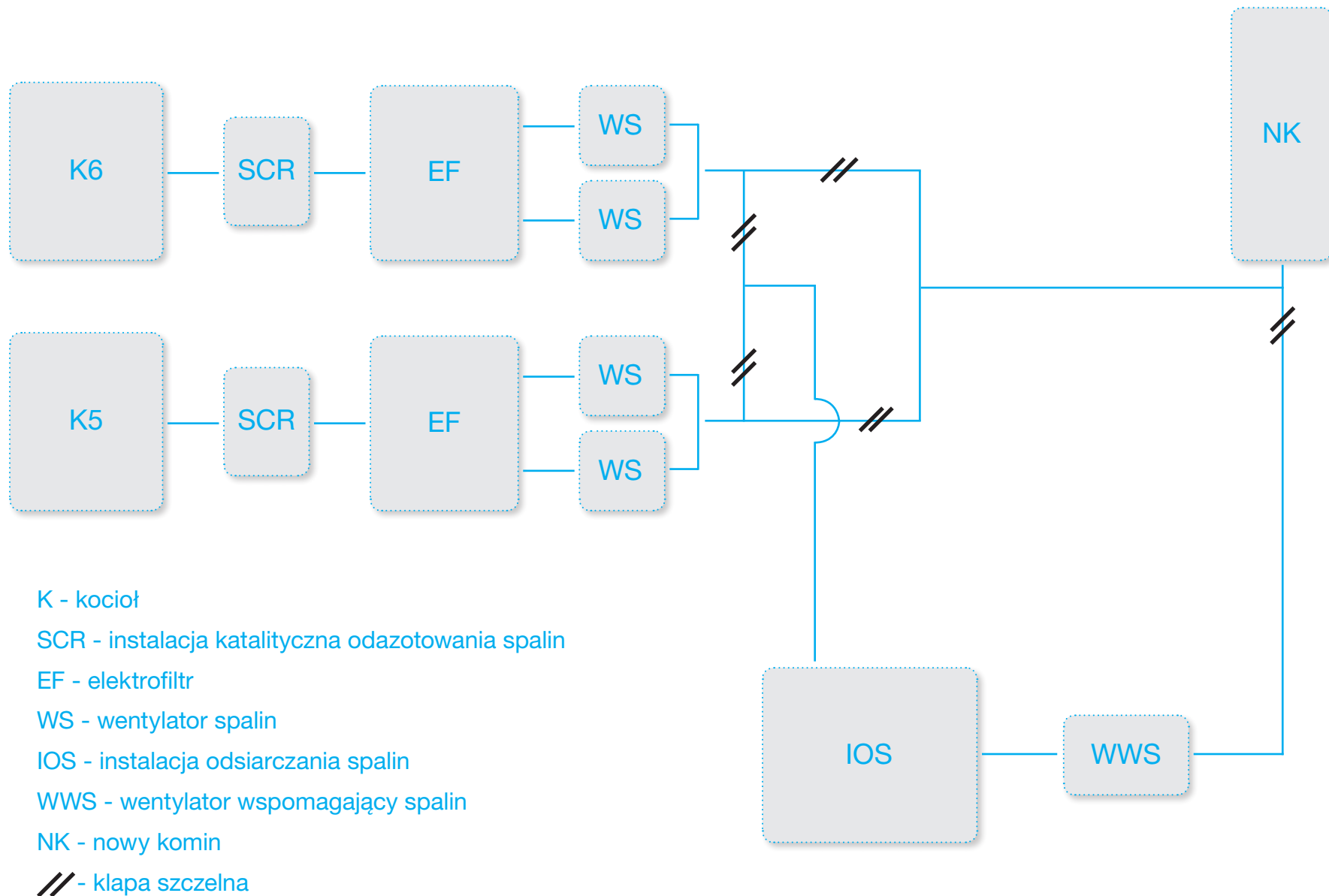
Ideowy schemat instalacji oczyszczania spalin w EC Elbląg
