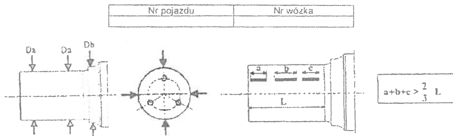
Załącznik 17 - Karta pomiarowa montażu łożysk maźniczych zestawu kołowego
