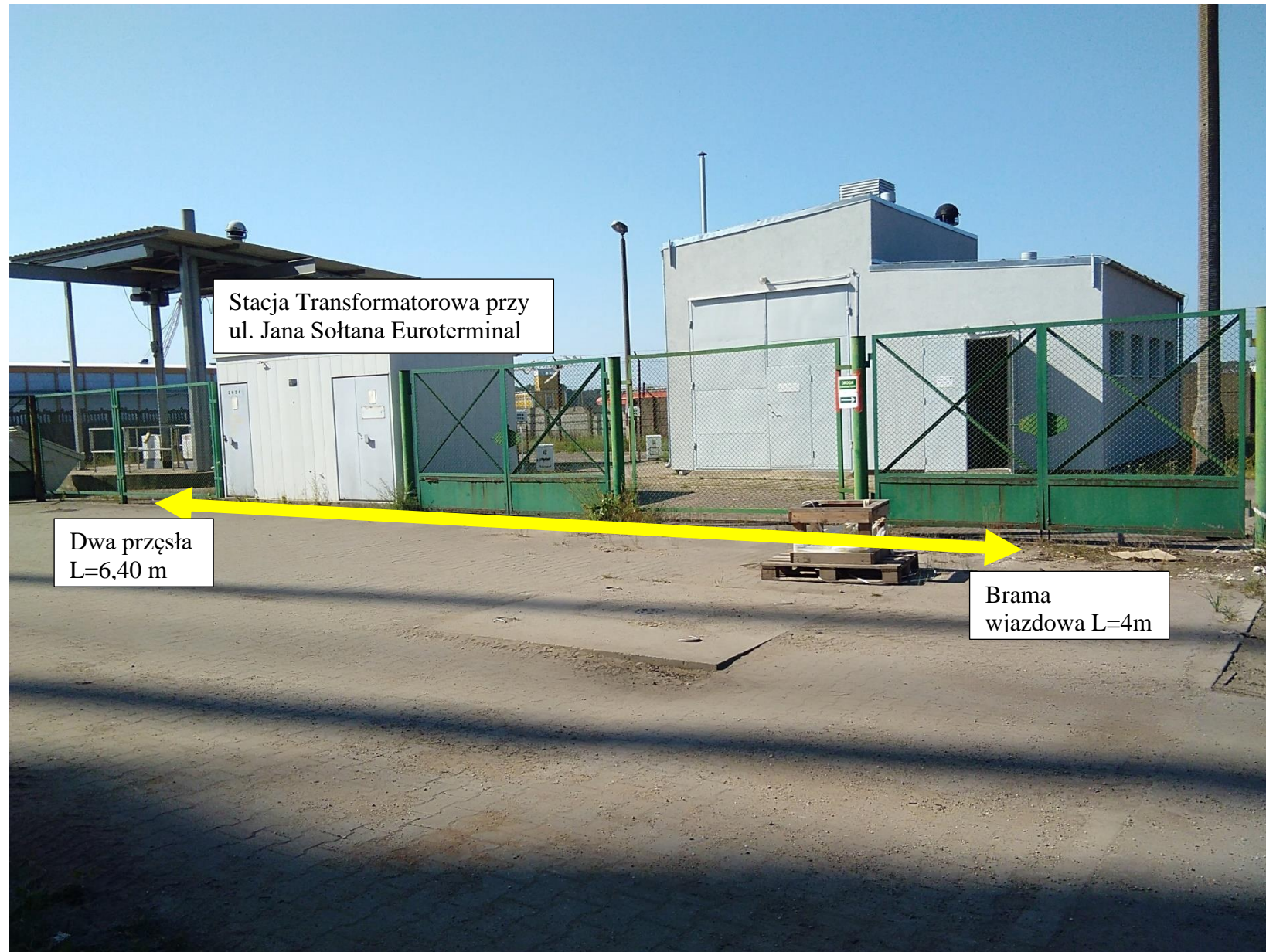
Zdj. nr 19. Ogrodzenie przy pompowni PP- zaznaczoną na zdj. bramę wjazdową należy wymontować i wstawić w miejsce przęseł z lewej strony stacji transformatorowej Zdemontowane przęsła należy wstawić w miejsce demontażu bramy.
