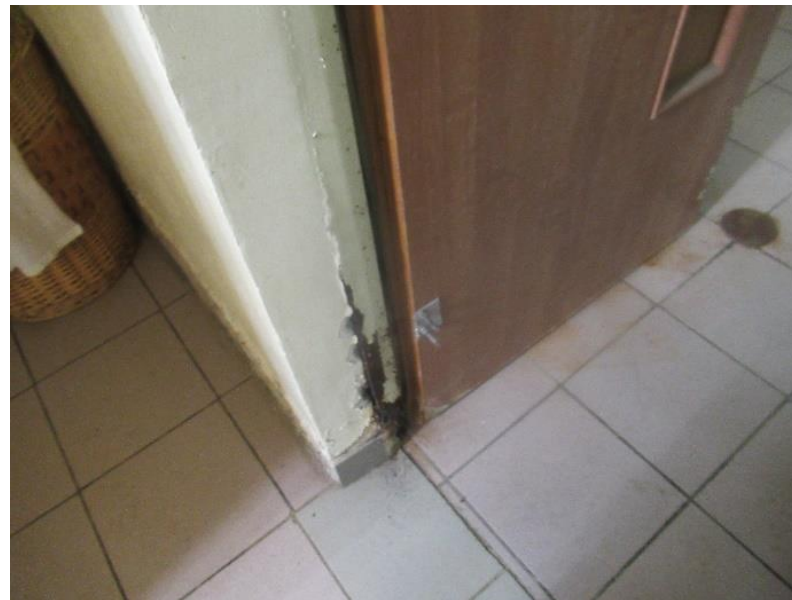
Zdj. nr 10. Pomieszczenie socjalne w pompowni P1 – wymienić drzwi wraz z ościeżnicą na aluminiowe.
