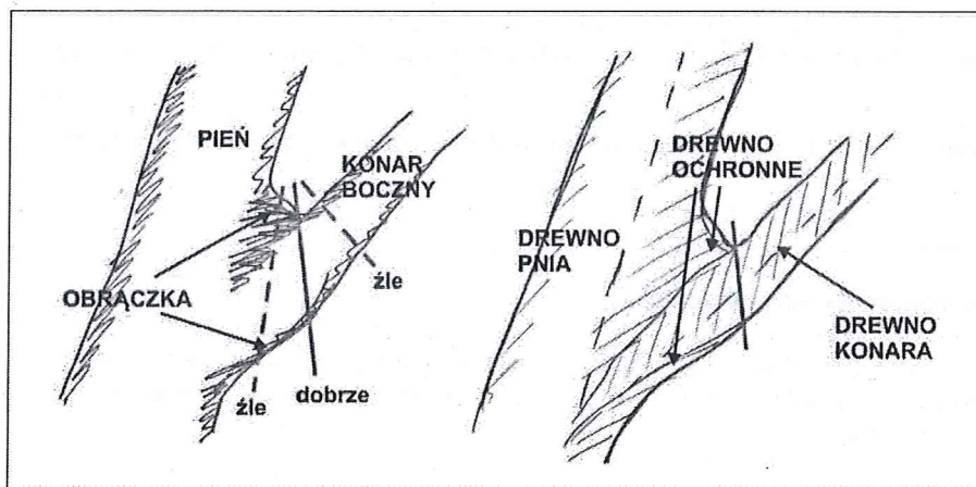
Rysunek nr 1 Schemat cięcia na tzw. „obrączkę”
