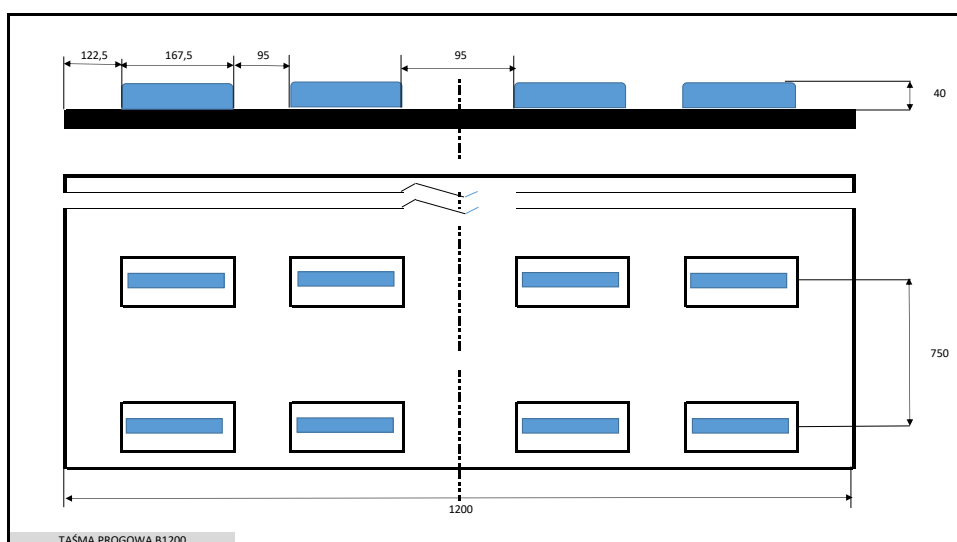
TAŚMA PROGOWA B1200
