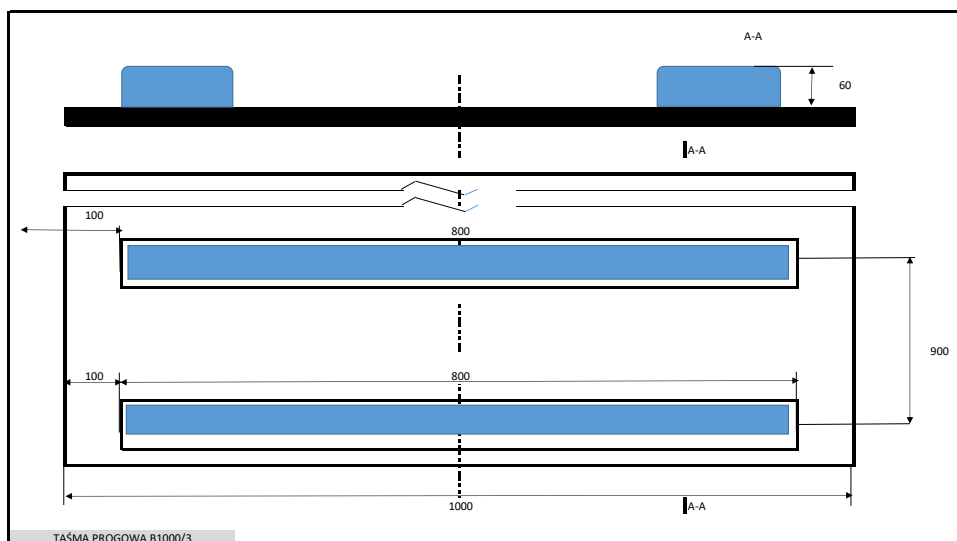
TAŚMA PROGOWA B1000/3
