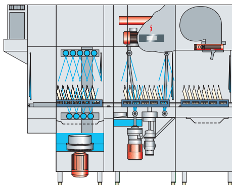
Widok przekrojowy zmywarki UPster® K-S 200
