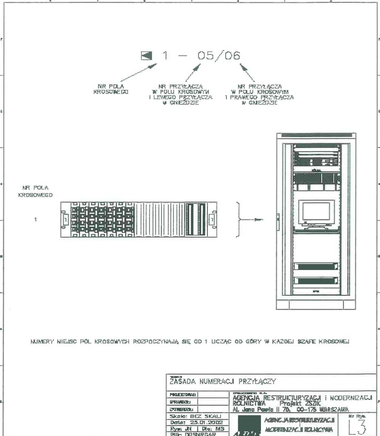
Rysunek 4: Zasada numeracji przyłączy - nr L3
