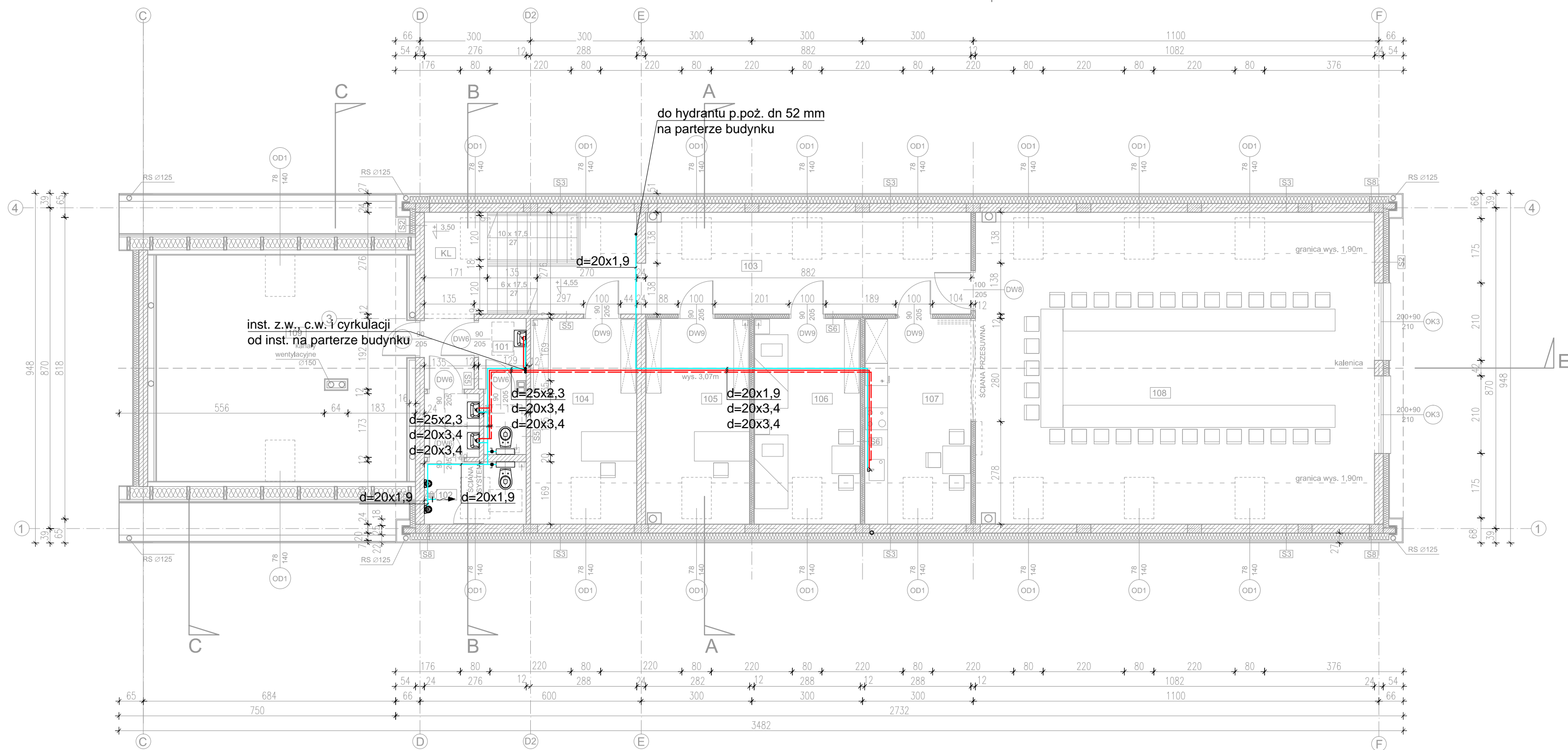
RZUT PIĘTRA BUDYNEK NOWY - CZĘŚĆ ROZBUDOWANA
