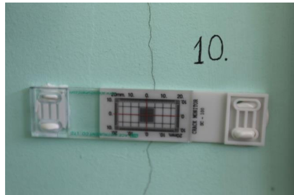
Szczelinomierz S10 – parter
