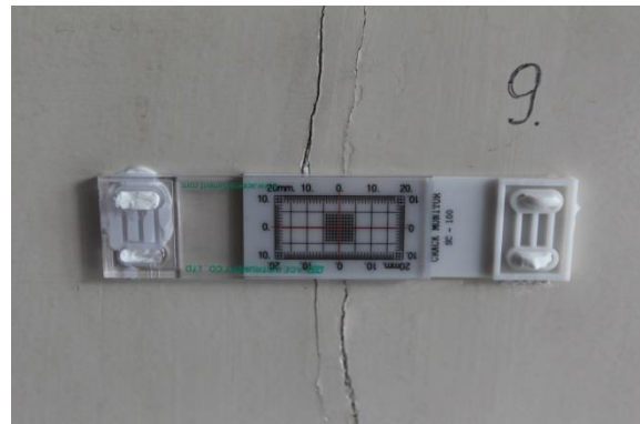
Szczelinomierz S9 – parter
