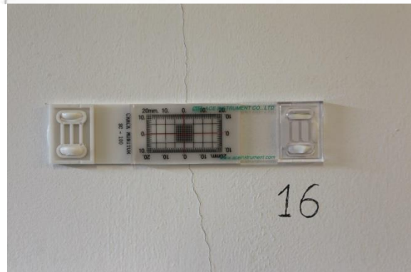
Szczelinomierz S16 – piwnica
