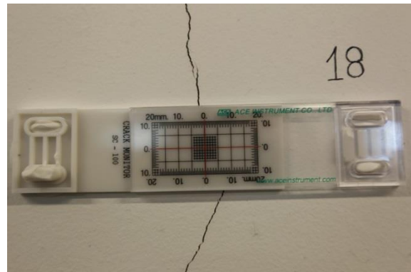
Szczelinomierz S18 – piwnica
