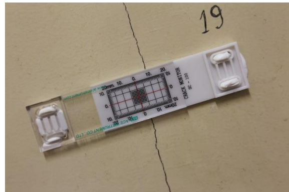
Szczelinomierz S19 – piwnica
