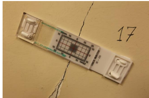
Szczelinomierz S17 – piwnica
