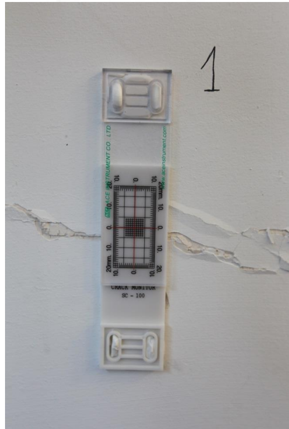
Szczelinomierz S1 – I piętro
