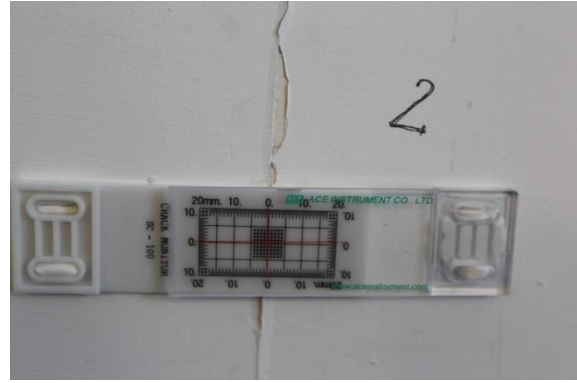
Szczelinomierz S2 – I piętro
