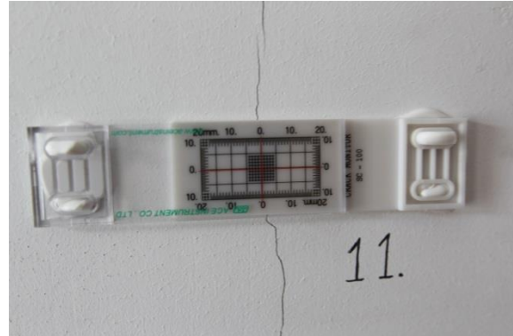
Szczelinomierz S11 – parter
