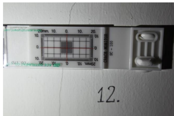
Szczelinomierz S12 – parter
