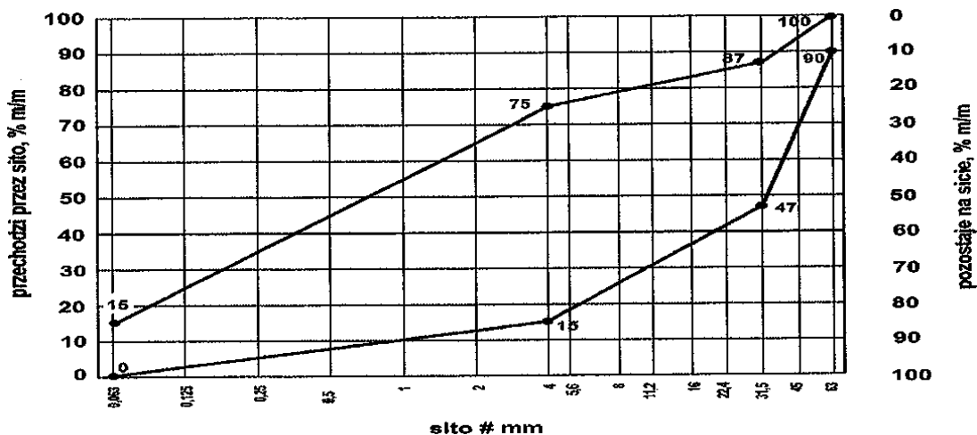
Rys. 7. Krzywe graniczne uziarnienia mieszanki kruszywa niezwiązanego 0/63 mm do nawierzchni. Mieszanki kruszyw niezwiązanych stosowane do nawierzchni z kruszywa niezwiązanego powinny spełniać wymagania wg tablicy 2. Wymagania wobec wrażliwości na mróz, mieszanek przeznaczonych do nawierzchni, dotyczą badania materiału po pięciokrotnym zagęszczeniu metodą Proctora według PN-EN 13286-2 [18]. Nie stawia się wymagań wobec wodoprzepuszczalności zagęszczonej mieszanki niezwiązanego do nawierzchni z kruszywa niezwiązanego, o ile szczegółowe rozwiązania tego nie przewidują.
