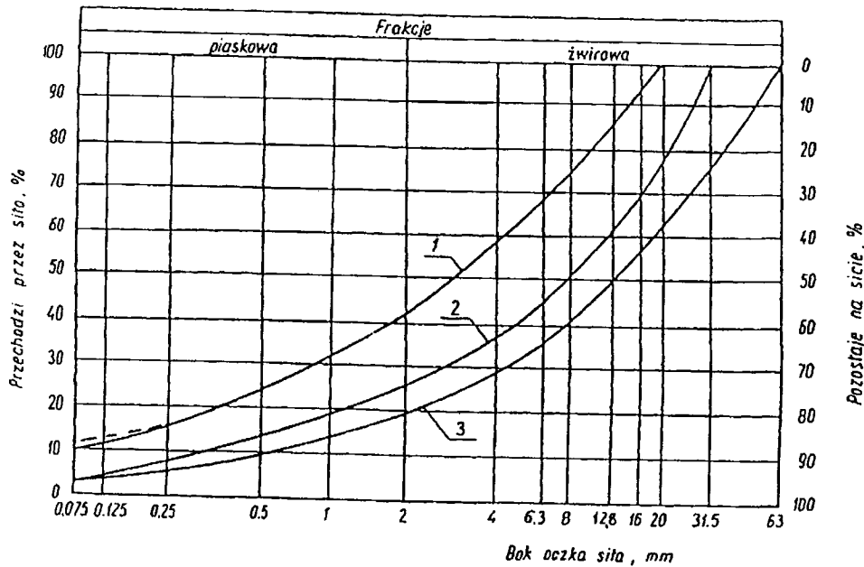
Rysunek 1. Pole dobrego uziarnienia kruszyw przeznaczonych na podbudowy stabilizowane mechanicznie 1-2 kruszywo na podbudowę zasadniczą (górną warstwę – nawierzchnię) lub podbudowę jednowarstwową 1-3 kruszywo na podbudowę pomocniczą (dolną warstwę)
