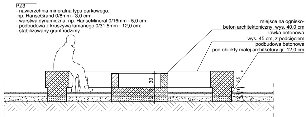
PRZEKRÓJ 1-1
