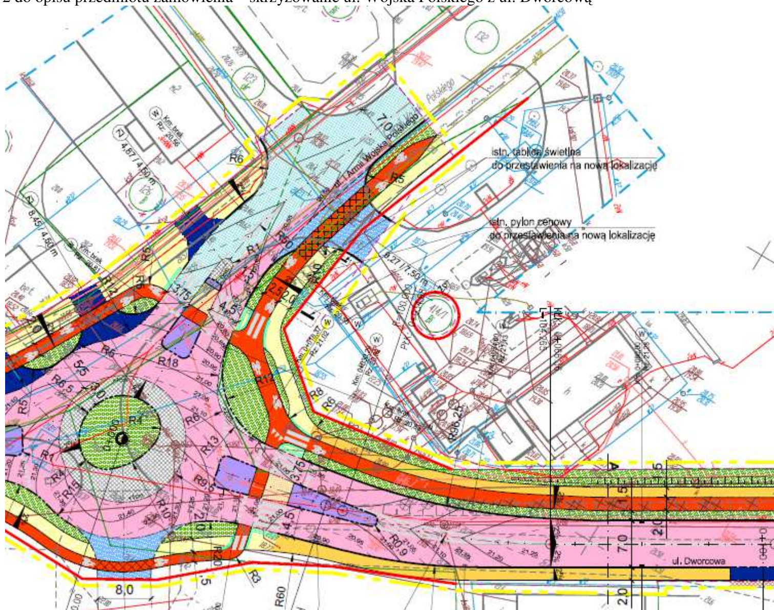
Załącznik nr 2 do opisu przedmiotu zamówienia – skrzyżowanie ul. Wojska Polskiego z ul. Dworcową
