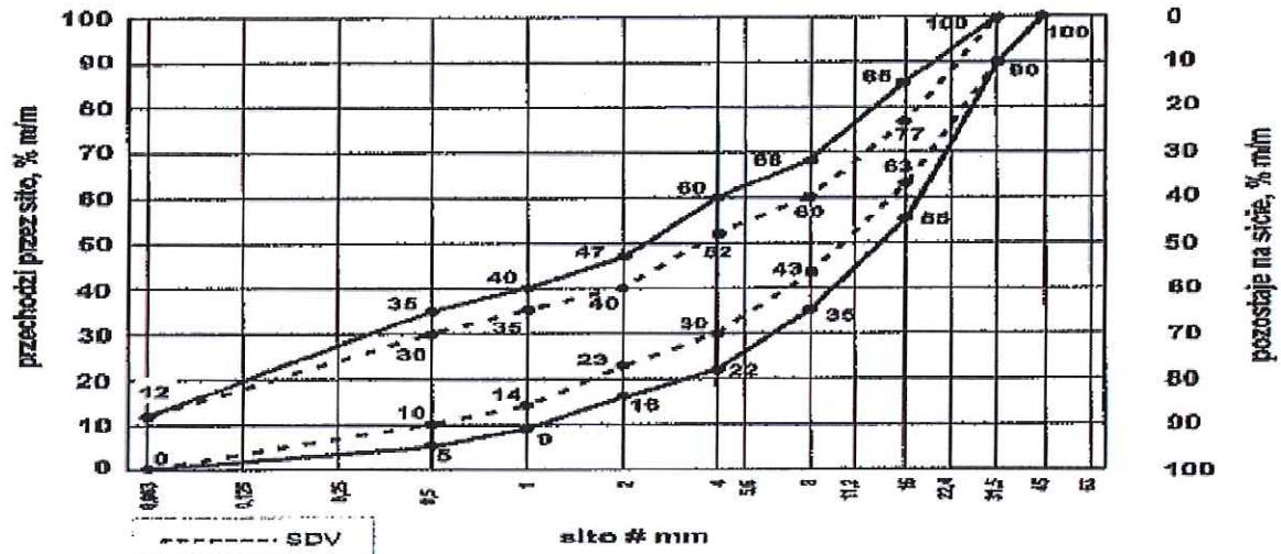
Rys. 1. Mieszanka niezwiązana 0/31,5 do warstw podbudowy pomocniczej Krzywa uziarnienia (S) /dla podbudowy zasadniczej/ powinna mieścić się w krzywych uziarnienia podanych na rys. 2 ograniczonych przerywanymi liniami (SDV) z uwzględnieniem dopuszczalnych tolerancji podanych w tablicy nr 2 oraz spełniać wymagania ciągłości uziarnienia zawarte w tablicy nr 3.
