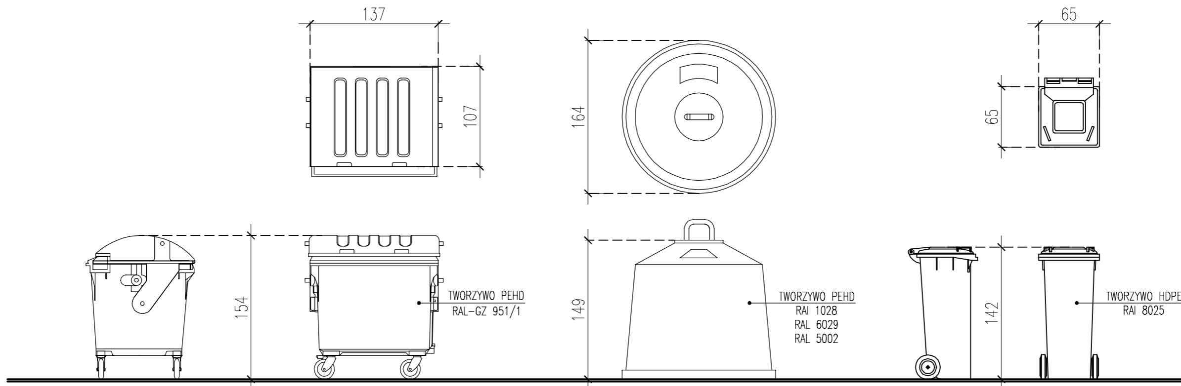
POJEMNIK NA ODPADY ZMIESZANE V = 1100L
