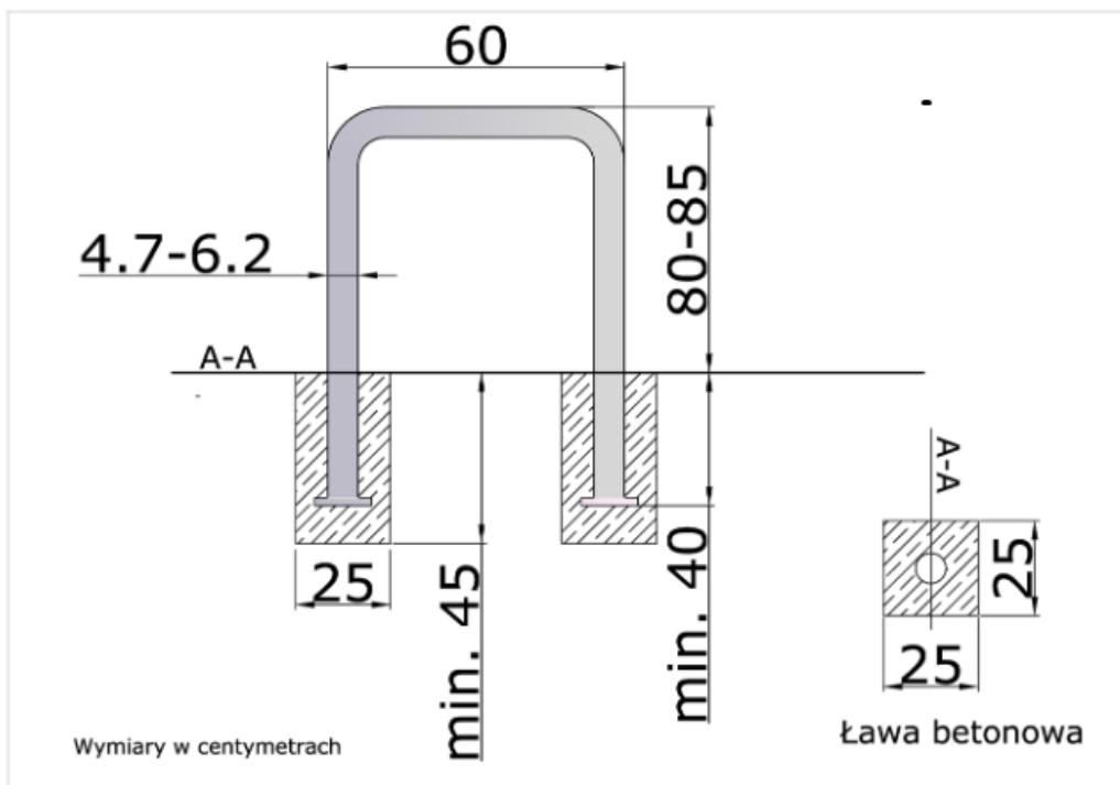
Rys. 26A. Stojak rekomendowany.
