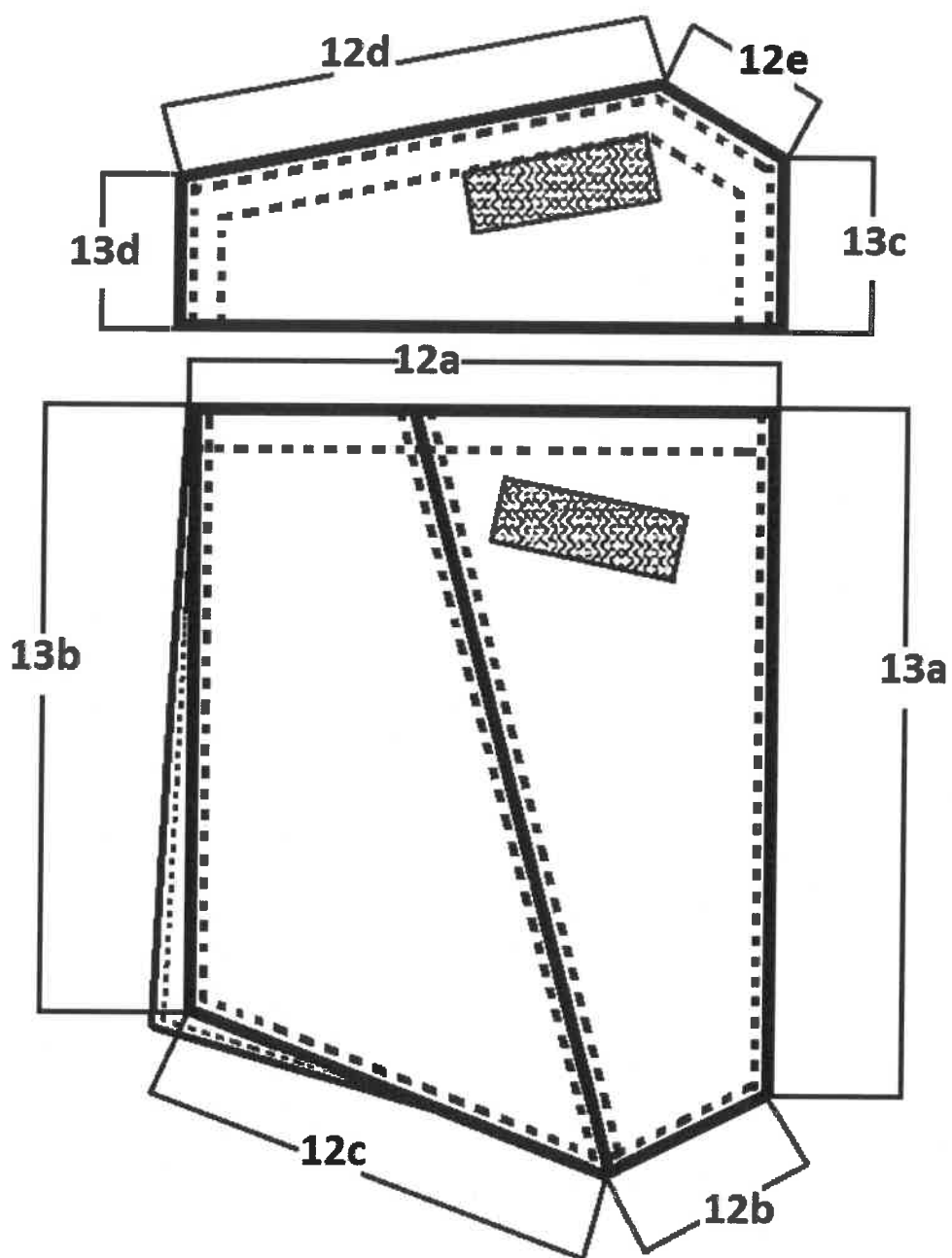
Rysunek 13 – Spodnie Kieszonka dolna
