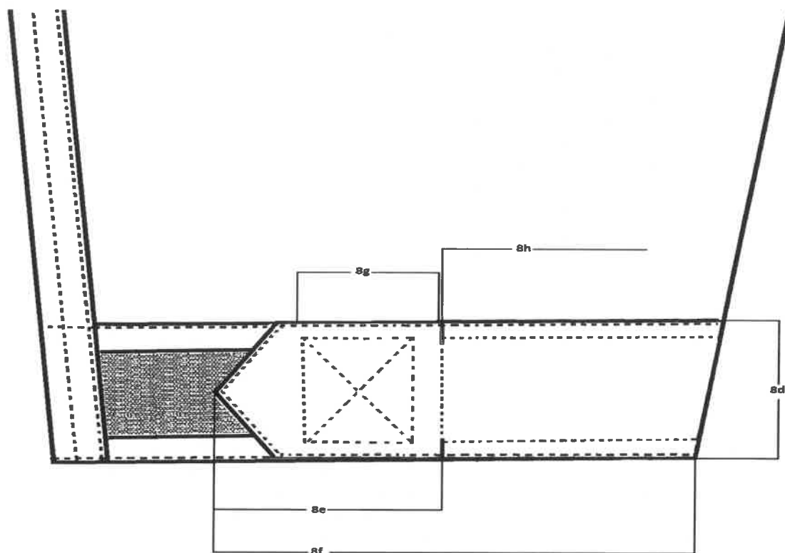
Rysunek 7 – dół rękawa lewego
